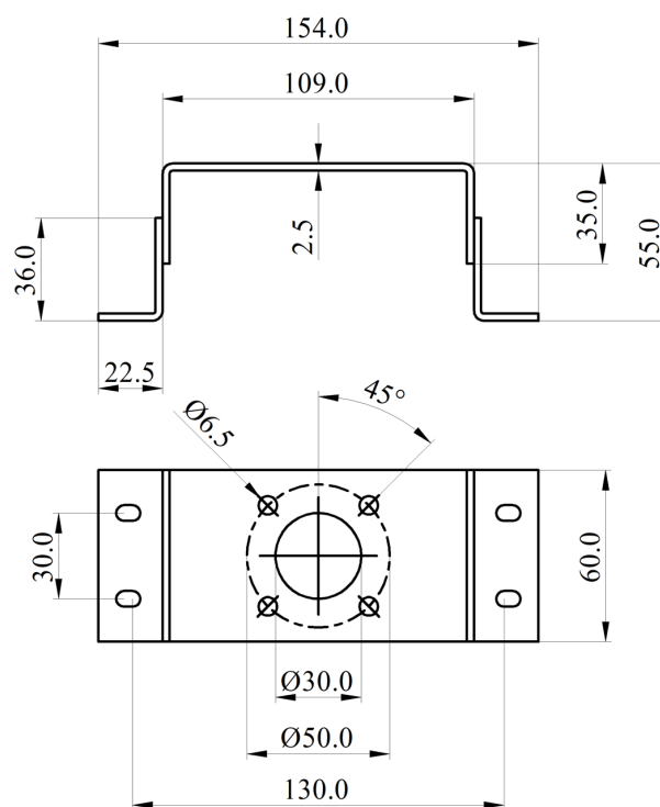
Монтажный кронштейн с угловым ходом в сборе, форма 2
