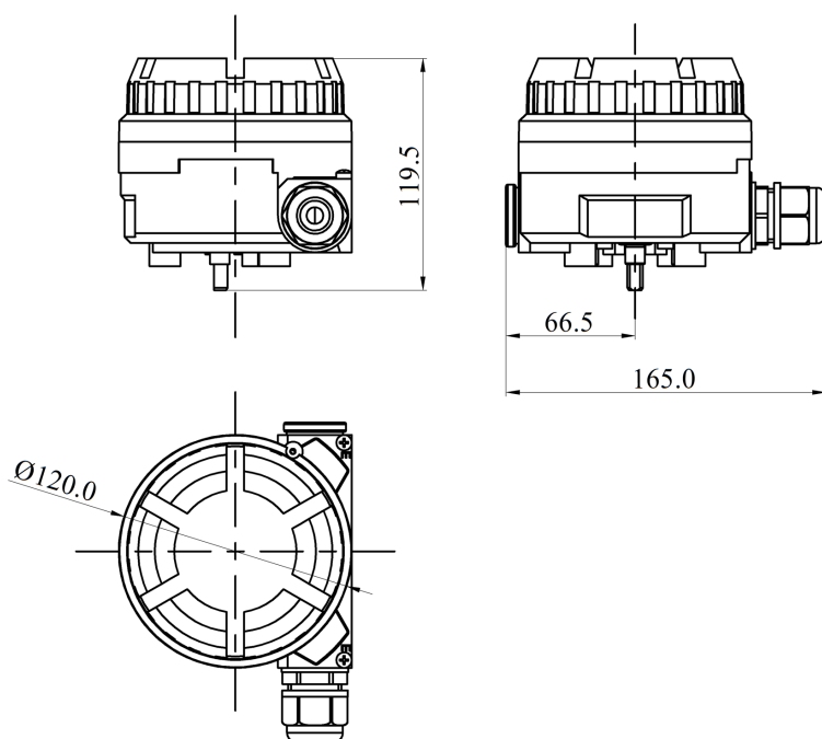
Размер удаленного датчика
