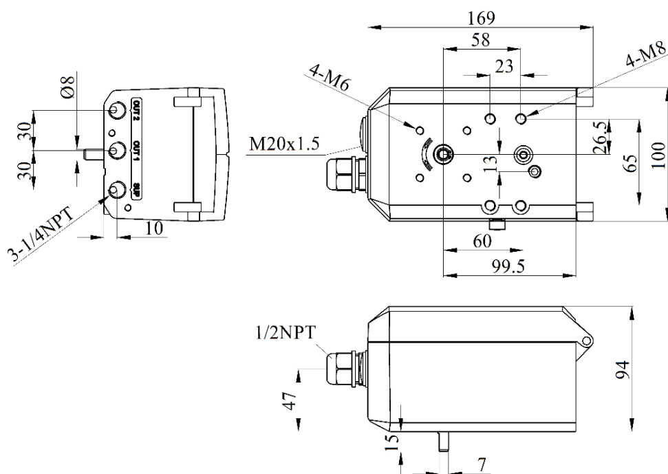
Механический размер стабилизатора
