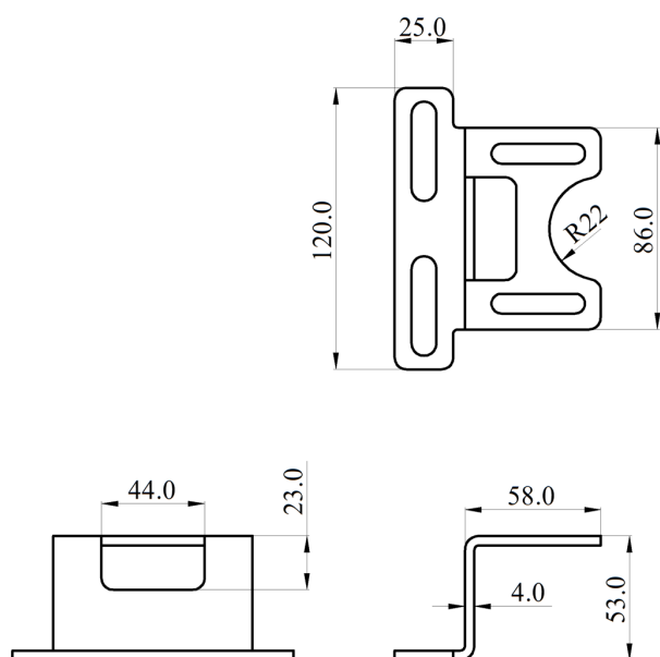
Монтажный кронштейн с прямым ходом
