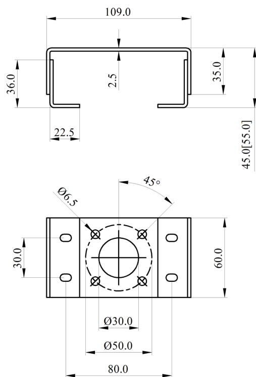
Монтажный кронштейн с угловым ходом в сборе, форма 1
