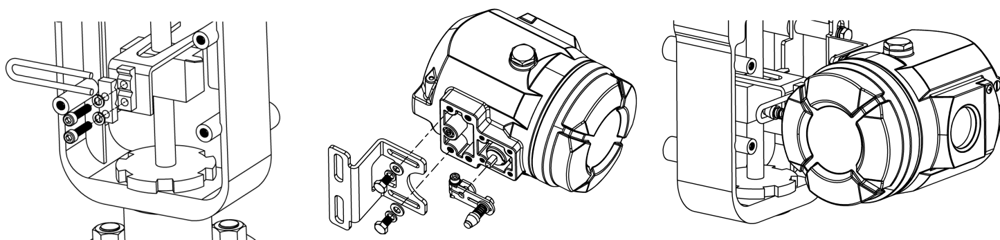
Искробезопасный прямой ход
