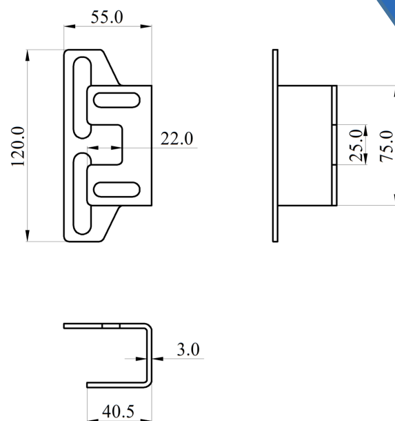
Монтажный кронштейн прямого хода с дистанционной передачей
