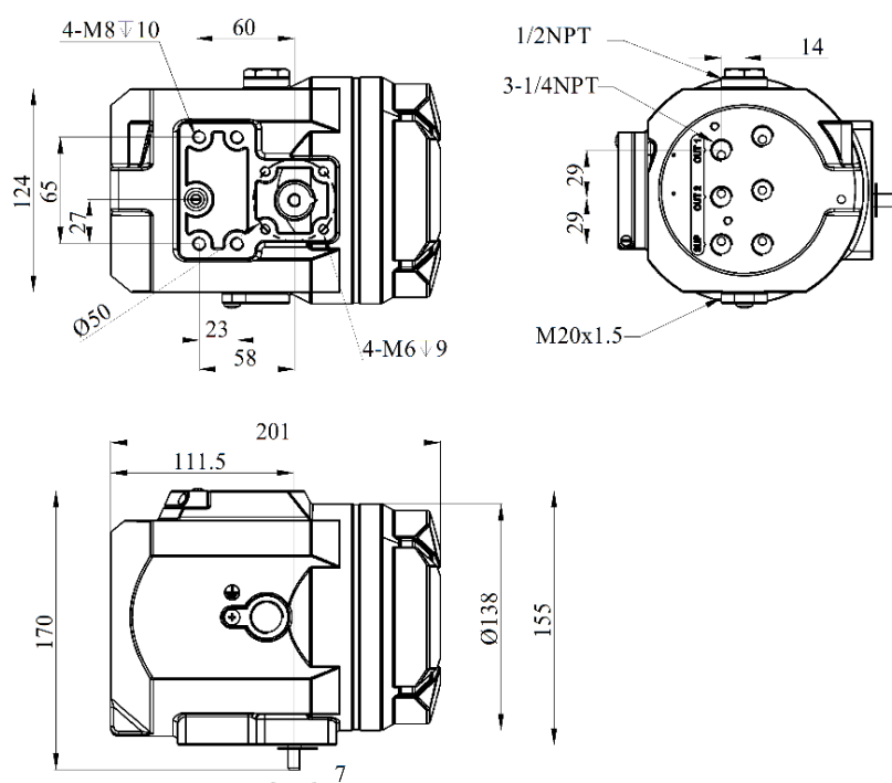
Механический размер огнестойкого позиционера
