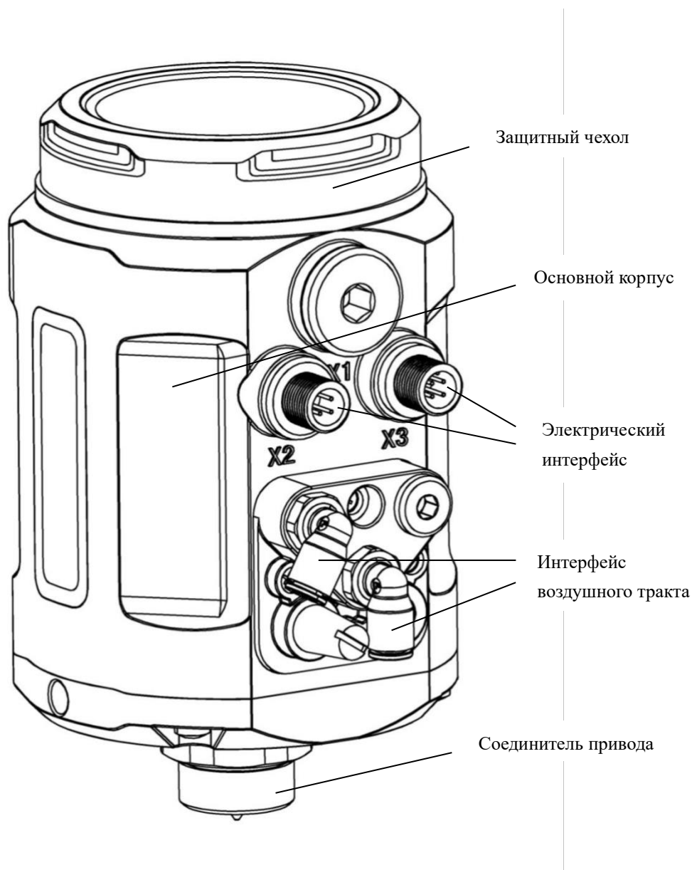
Изображение 1. Структура позиционера
