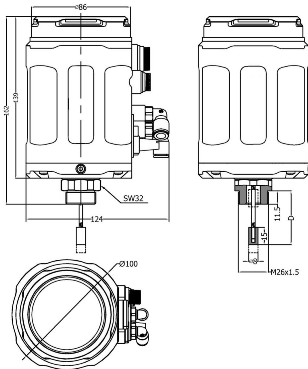
Изображение 3. Размеры прямого хода
